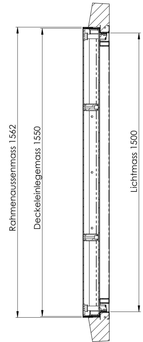
SCHNITT B-B MABSTAB 1 : 10
